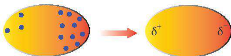
▲ Hình 11.7. Lượng cực tạm thời được hình thành do sự phân bố không đồng đều của các electron trong phân tử
