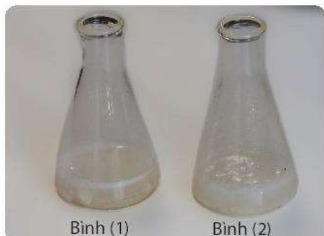
▲ Hình 16.6. Minh hoạ thí nghiệm nghiên cứu ảnh hưởng của bề mặt tiếp xúc đến tốc độ phản ứng
