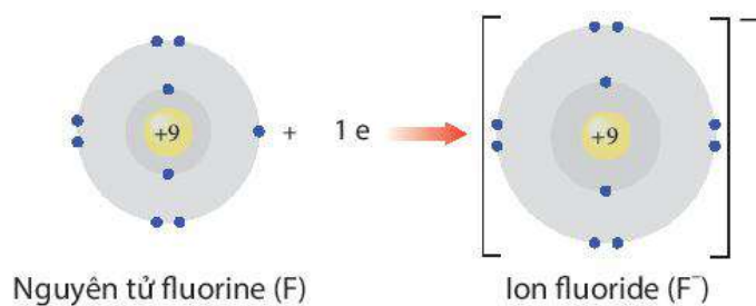
▲ Hình 8.4. Sự hình thành ion F^-
