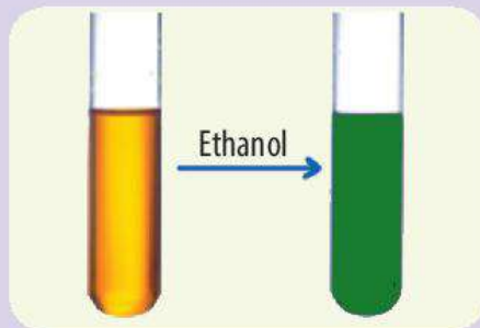
▲ Sự chuyển màu từ da cam ( \text{Cr}_2\text{O}_7^{2-} ) sang xanh ( \text{Cr}^{3+} )
