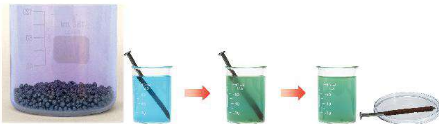
(a) Quá trình thăng hoa của iodine (b) Nhúng đinh sắt vào dung dịch copper sulfate
