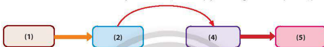
Sơ đồ các bước nghiên cứu hoá học
