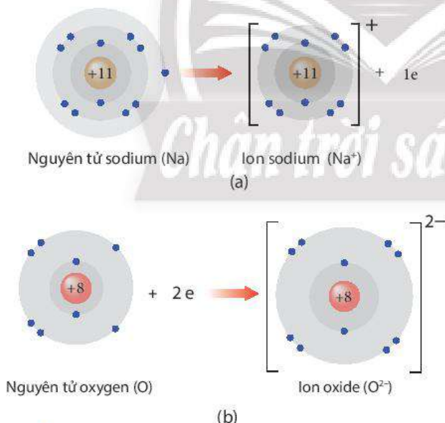
▲ Hình 9.1. Minh hoạ quá trình hình thành ion
