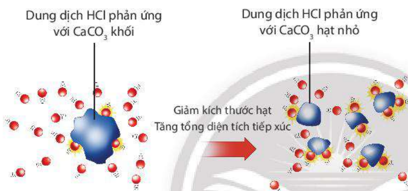
▲ Hình 16.7. Minh hoạ dung dịch HCl phản ứng với \text{CaCO}_3 có kích thước khác nhau
