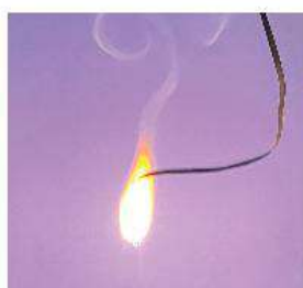
▲ Hình 12.1. Magnesium phản ứng với oxygen
