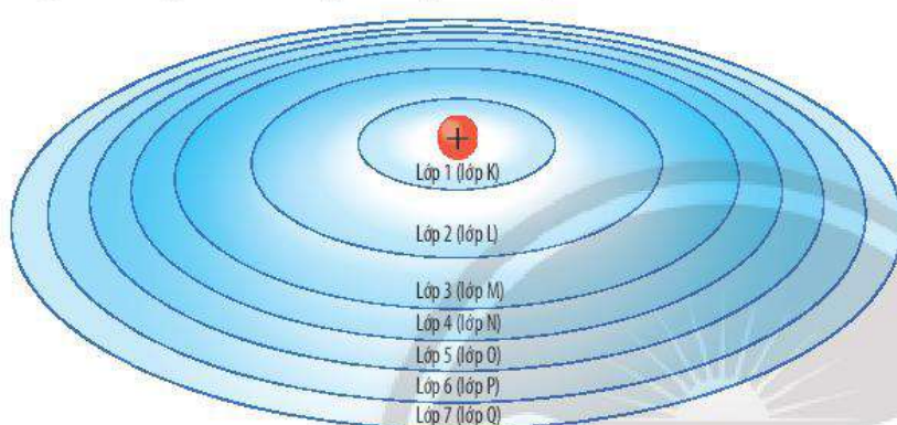
▲ Hình 4.5. Minh họa các lớp electron ở vỏ nguyên tử
